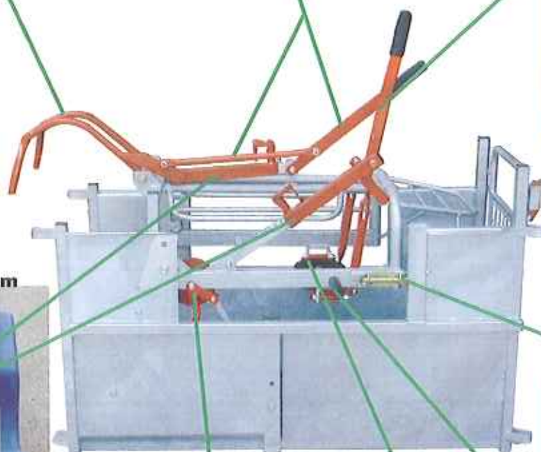
Vérin 350
